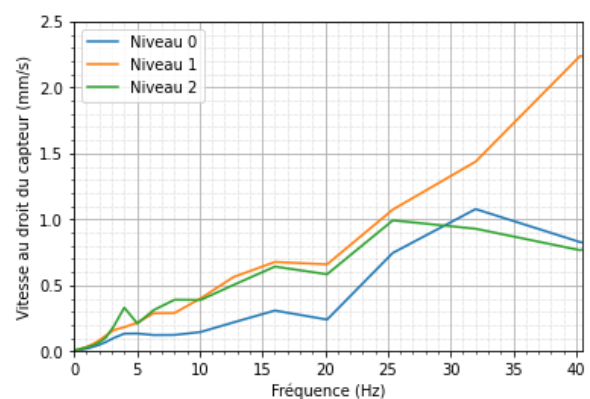
Figure 11 : Vitesses calculées à l'emplacement du capteur C4 pour les trois niveaux de modélisation sous un chargement harmonique unitaire (1 MN)
