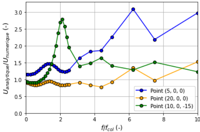
Figure 9: Rapport \bar{U} en fonction de la fréquence pour trois points du massif tricouche ( G = 50 MPa)
