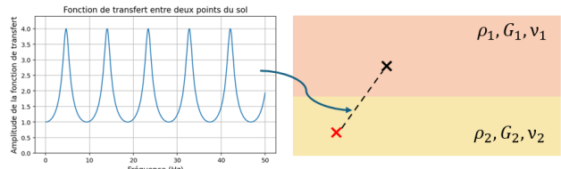
Figure 5 : Exemple d'amplification mesurée entre deux points du massif en fonction de la fréquence
