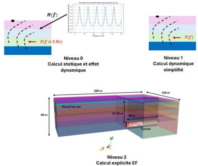
Figure 10: Niveaux de modélisation
