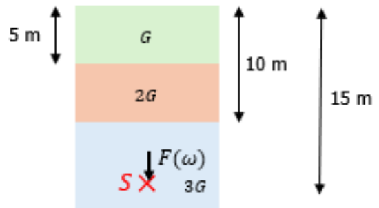
Figure 8: Schéma de la configuration tricouche étudiée
