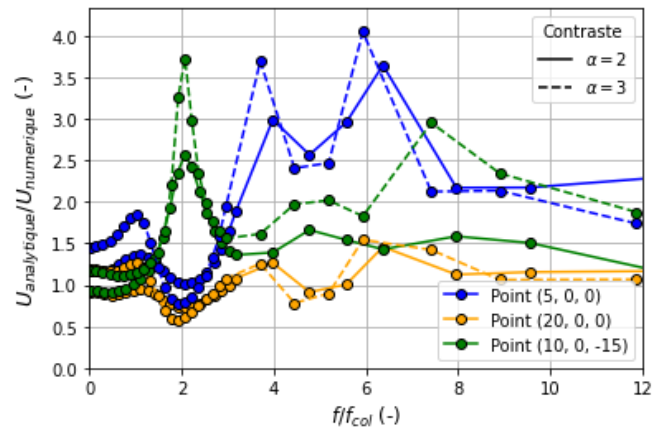
Figure 7 : Rapport \bar{U} en fonction de la fréquence pour trois points du massif bicouche ( G = 50 MPa)
