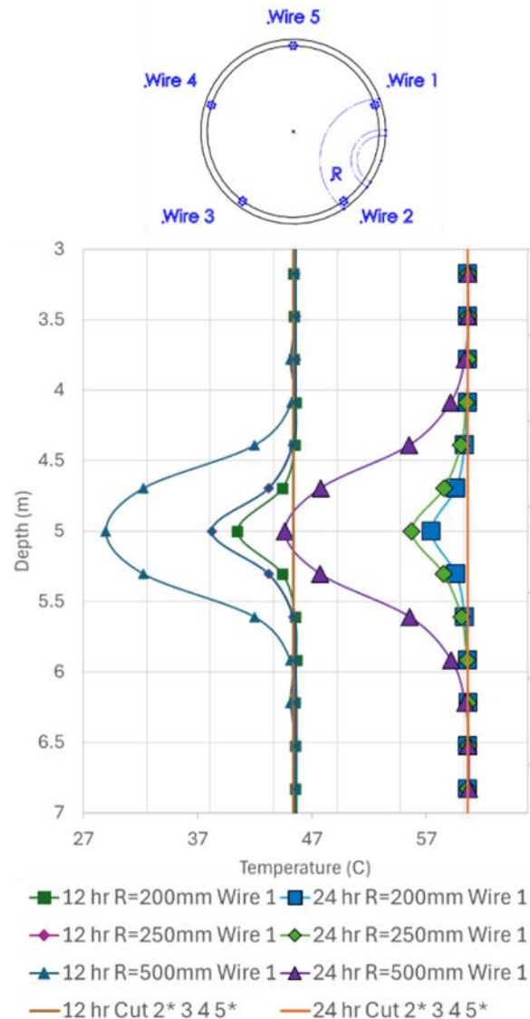
Figure 5. Températures obtenues du modèle numérique avec inclusion sphérique sableuse au milieu de 2 chaînes thermiques (adapté de Baudo,2024)
